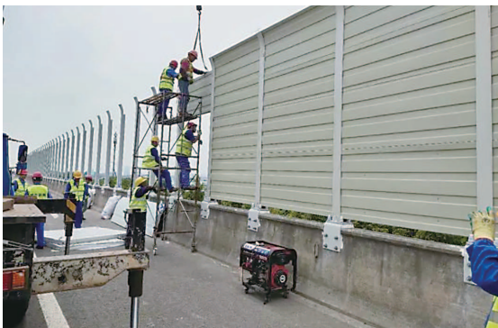
S32申嘉湖高速安装隔音屏
